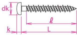
プラグレスアンカー (ナベ頭)
