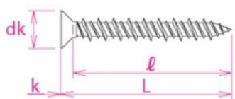
プラグレスアンカー (皿頭)
